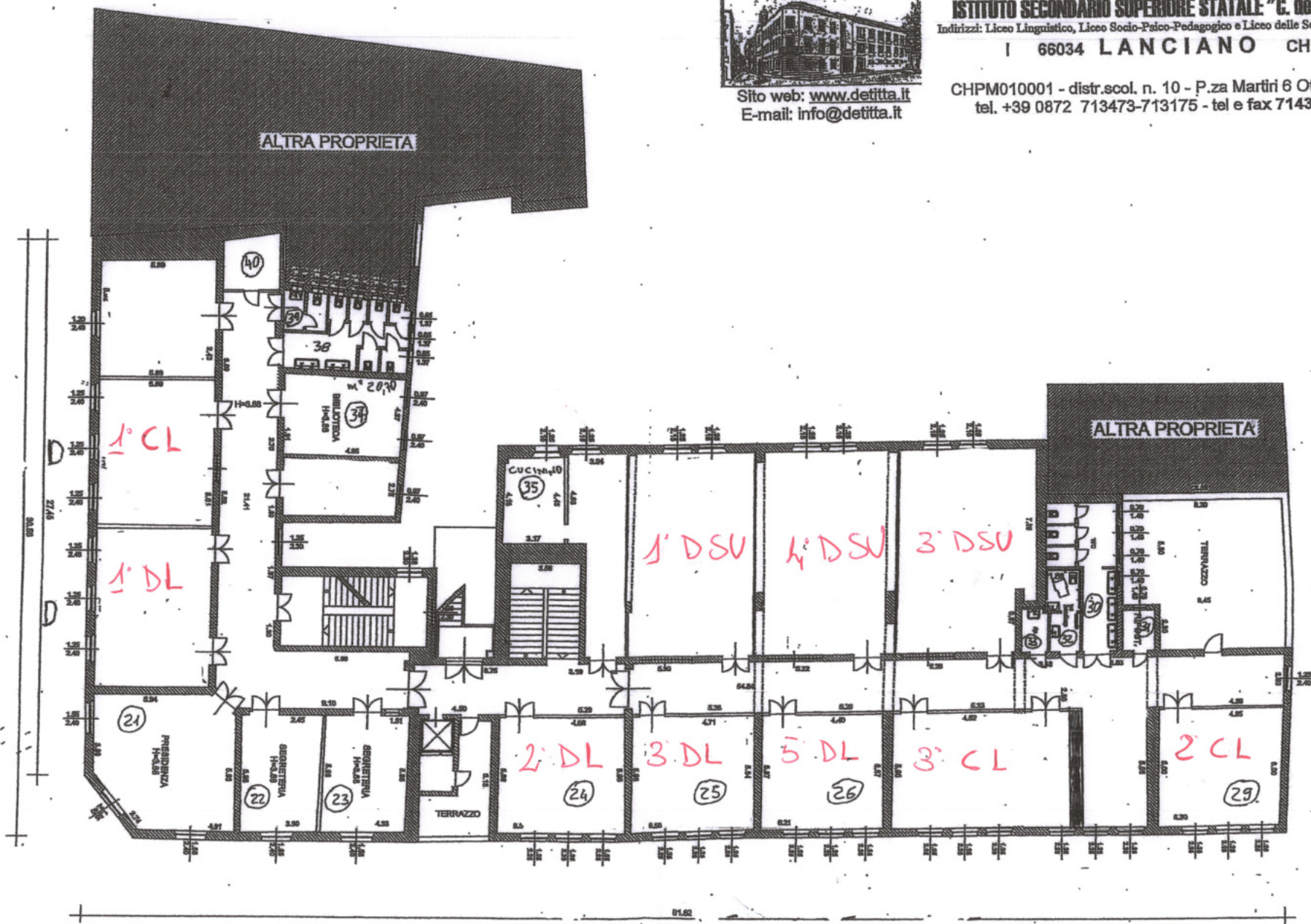
Pianta P.1° scala 1:200
